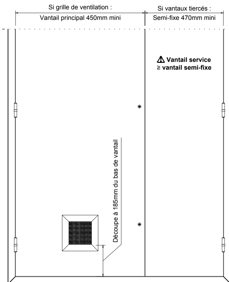
Position de la grille de ventilation sur un bloc-gaine standard
