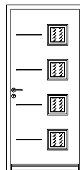
Linéa Zen 4CV U_g=1.4 (HB) U_g=1.7 (HM)
