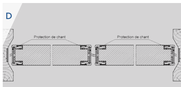
D : Plan protections de chants pour bloc-porte double action Pour plus d'information, cf. MBO-016
